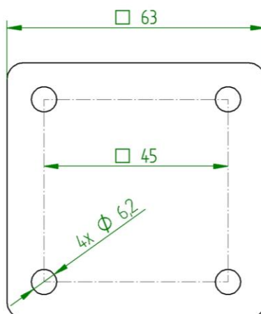
Nákres upevnění svítidla:
